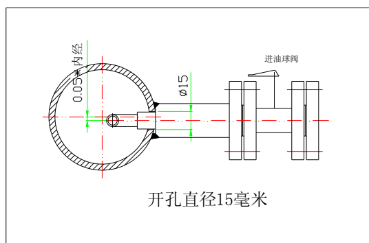
零压安装用探头焊接组件
