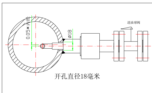
带压安装用探头焊接组件
