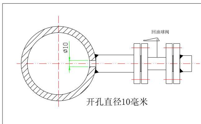
回油焊接组件
